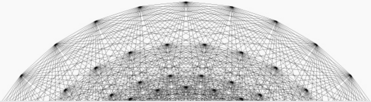
Figura 4: El politopo 421 es la forma algebraica en el centro de una teoría universal de todo. La teoría es un intento de reconciliar uno de los problemas no resueltos de la física: la unificación de la física cuántica y la gravitación con la esperanza de explicar la estructura del universo. Este modelo, dibujado a mano en Illustrator fue diseñado por Peter Crnokrak en 2010.
