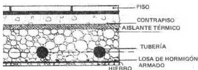
Fig.6. Losa radiante de techo. 24
