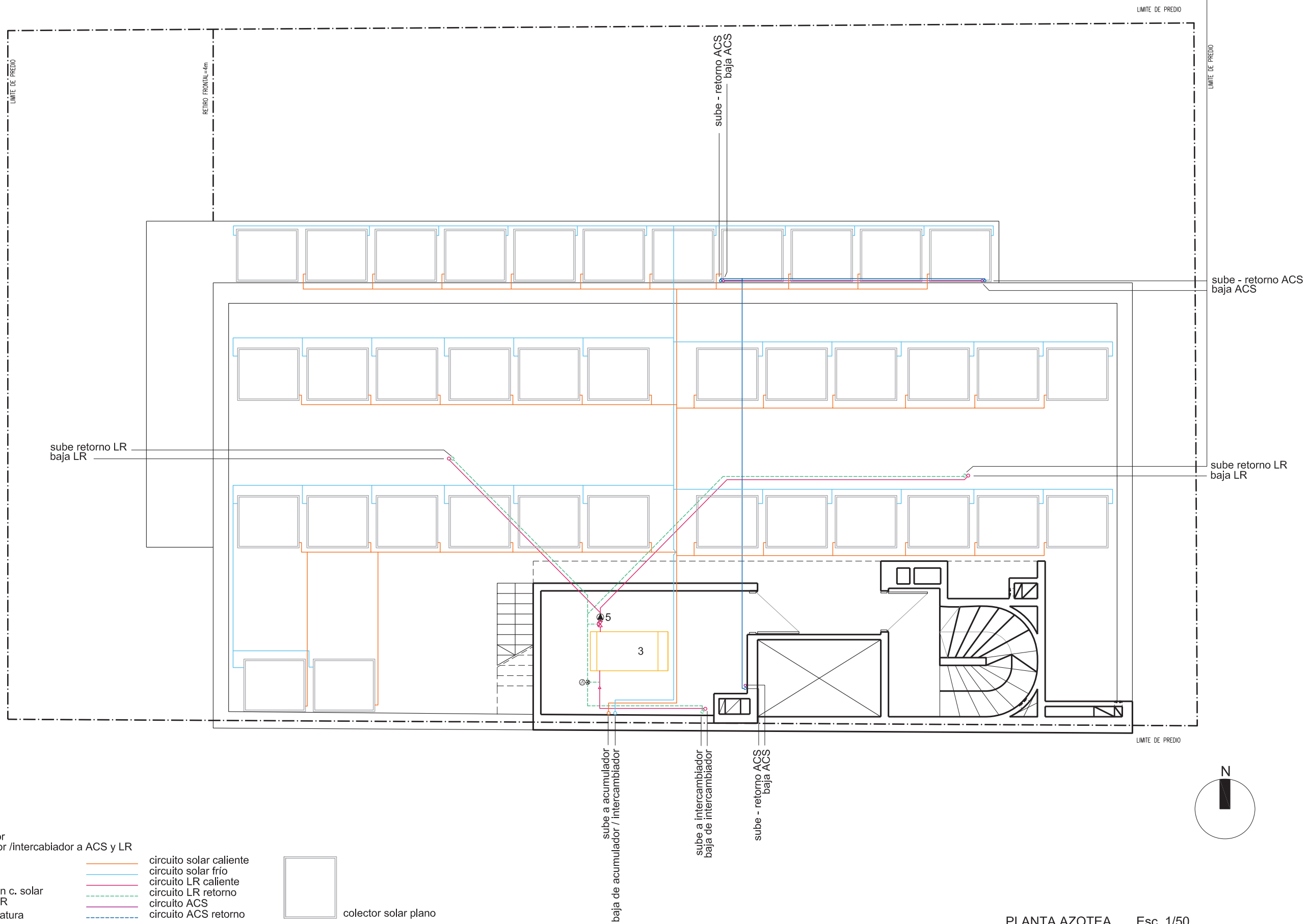
PLANTA AZOTEA . Esc. 1/50
