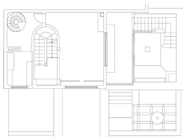
Vilamajó - Área 59 m2 (nivel +5.585) y Área 58 m2 (+11.085)
