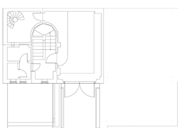
Vilamajó - Área 59 m2 (nivel 0.00) y Área 60 m2 (+2.785)
