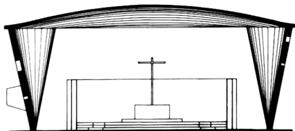
sección transversal
