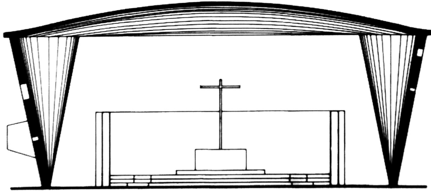
sección transversal
