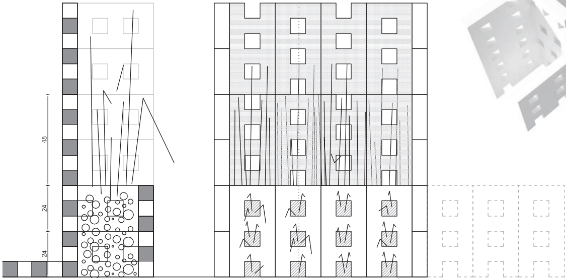
SECCIÓN 01
