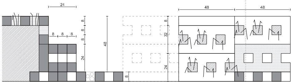
SECCIÓN 01
