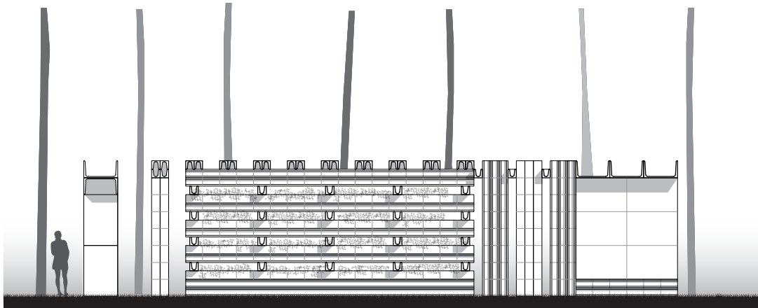
Fachada oeste esc. 1/125
