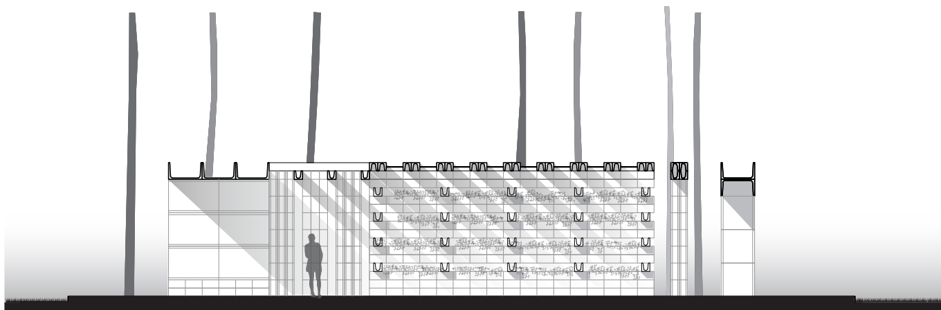
Corte A-A esc. 1/125
