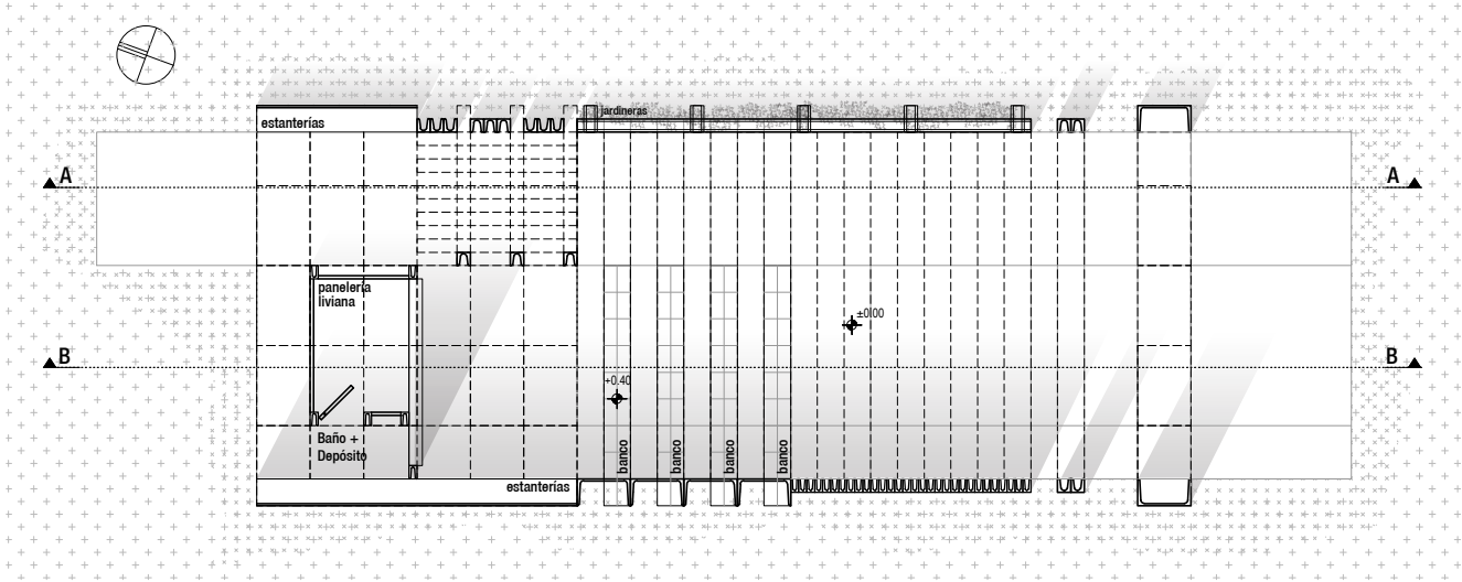
Planta esc. 1/125
