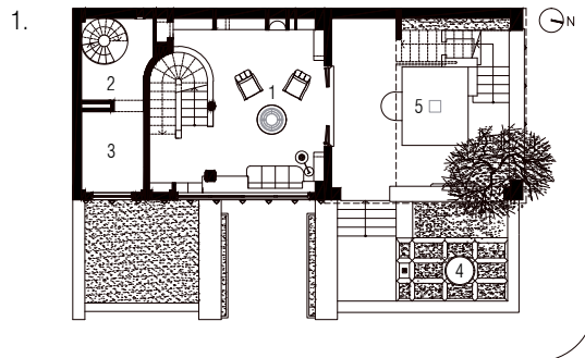
1- Living 2- Circulación de servicio 3- Dormitorio de servicio 4- Jardín elevado 5- Terraza
