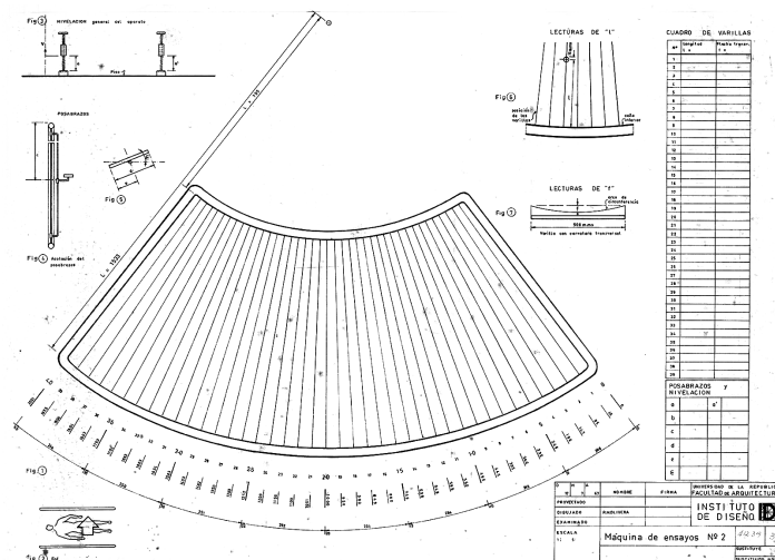
▲ Lámina inferior: Máquina de ensayos N°2. IdD. Lámina sup. Verificador de superficies de apoyo. IdD.
