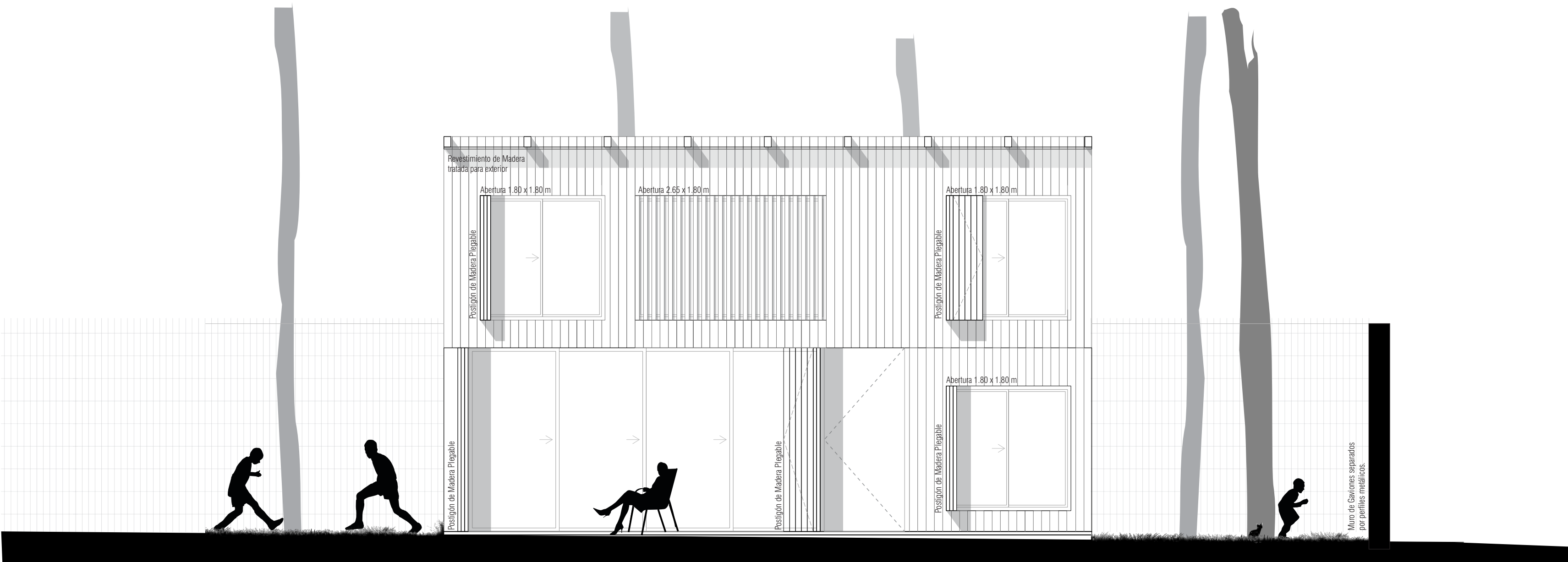
FACHADA LATERAL esc 1.50
