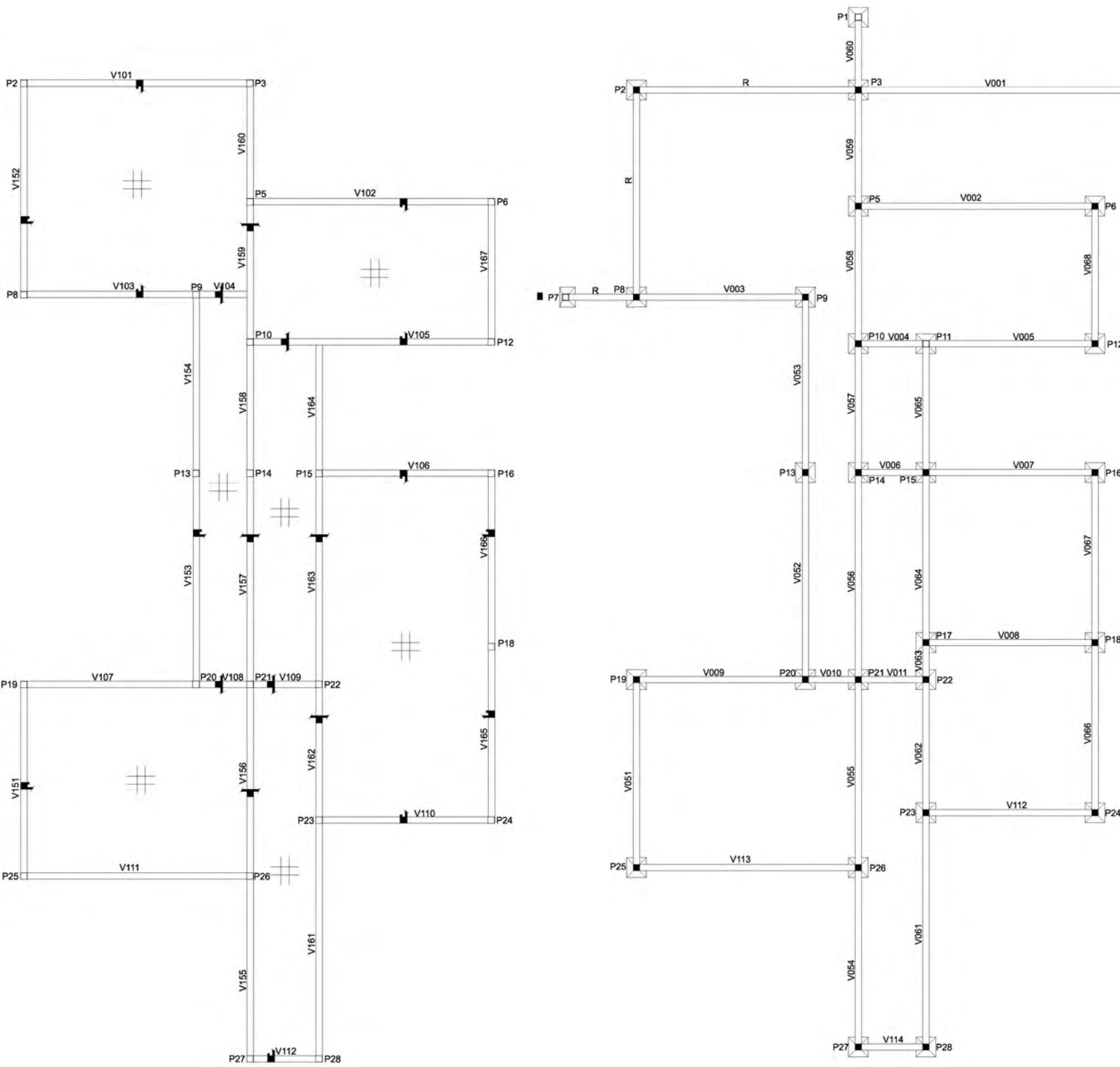
Esquema estructura de cubierta
